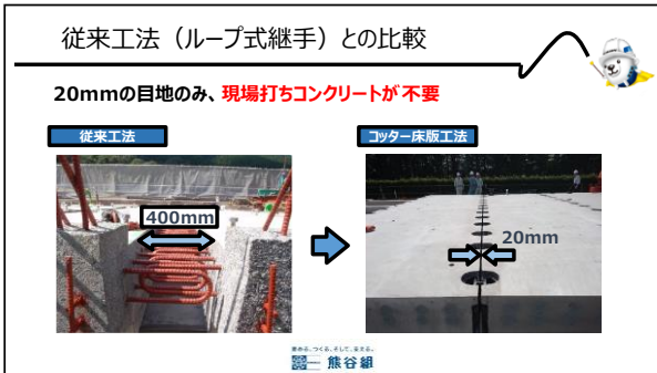
従来工法(ループ式継手)とコッター継手との比較
