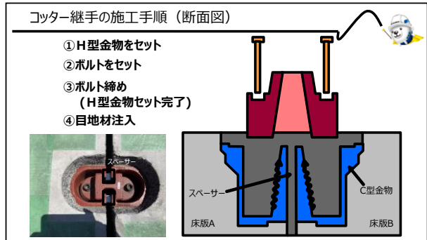
コッター継手の施工手順
