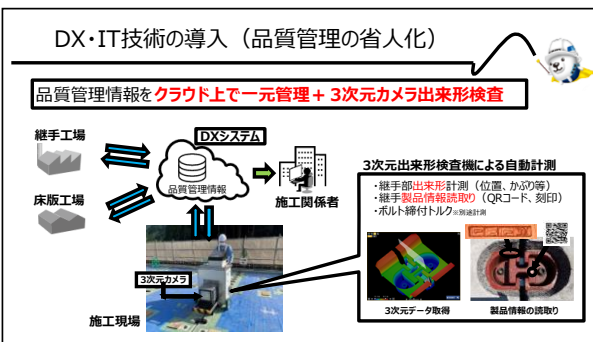
DX・IT技術の導入(品質管理の省人化)
